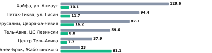
Пиковые NOx на транспортных станциях, ppb: канун Йом-Кипура и день Йом-Кипура
